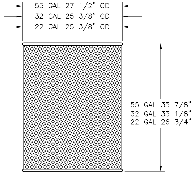
RECEPTACLE DIMENSIONS
